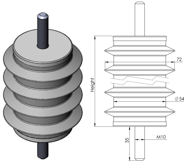
مشخصات ابعادی برقی SVL
